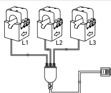
Stromwandler (×3)
